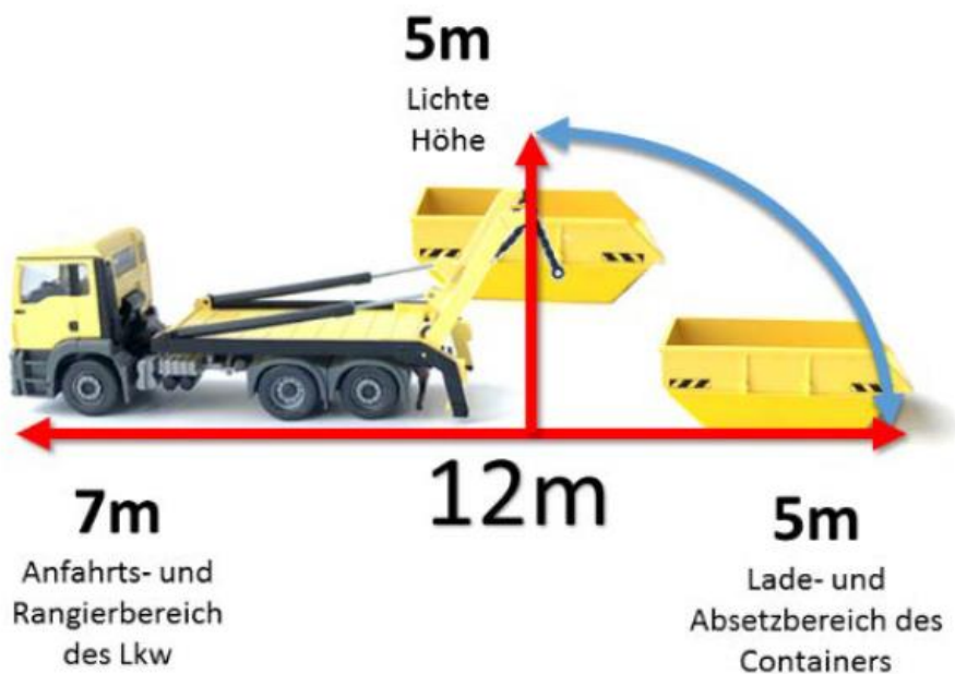
Absetzkipperfahrzeug mit Absetzbehälter
