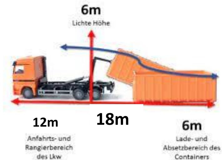
Abrollcontainerfahrzeug mit Abrollbehälter
